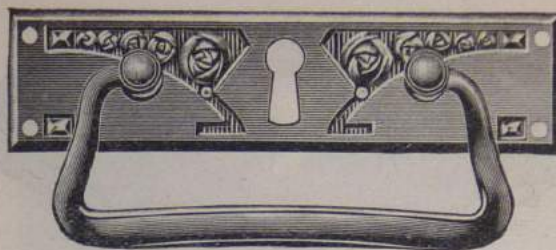
Handtag av blankpolerad mässing N:o 451. Utan nyckelhål. Längd 97 mm. » 0451. Med » » 97 »
