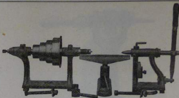
N:o 2. Träsvarvbeslag
