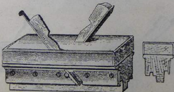
N:o 122. Spänt- och Nothyvlar, med järn
