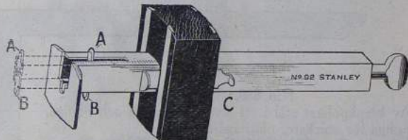
N:o 92. Amerikanskt Ritsmått »Stanley» Anslaget av rosenträ, m. mässingsbeslag. Stången av mässing, graderat i mm. Även avsett för dörr- o. fönstergångjärn. Längd 16½ cm.
