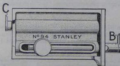
N:o 94. Amerikanskt Ritsmått »Stanley» Av stål, fint förnicklat. Graderat i mm. Speciellt avsett för dörr- och fönstergångjärn etc. Längd 7½ cm.
