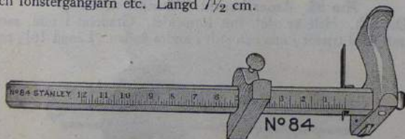
N:o 84. Amerikanskt Ritsmått »Stanley» Detta mått är försett med valslager samt ett stort handtag. Kniven är av stål och justerbar. Anslaget kan med en skruv fastsättas för det avstånd som önskas. Stocken är graderad upp till 12 tum. Tillverkat av bok. Längd 43 cm.
