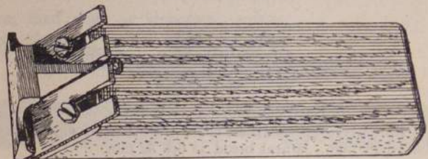
N:o 1181. Simshyvel (s. k. »groda»)
