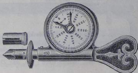
Slagtäljare
