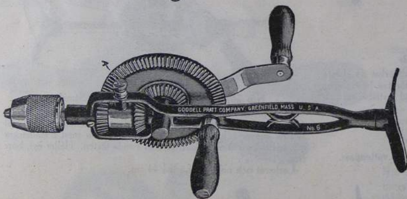
N:o 245. Amerikanskt Bröstdorr
