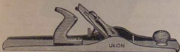
Amerikanska Rubankar »Union», med dubbla järn
