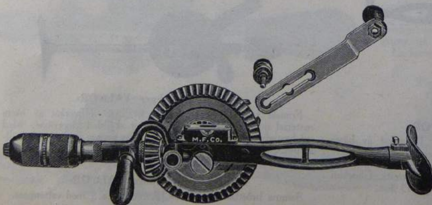
N:o 12. Amerikanskt Bröstdorr
