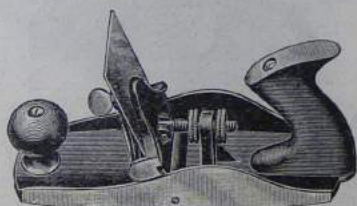
N:o 0112. Fanérhyvel »Kunz», med järn
