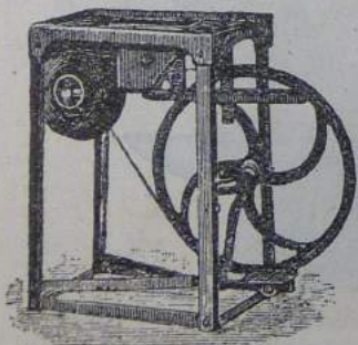
N:o 113. Fältässjor
