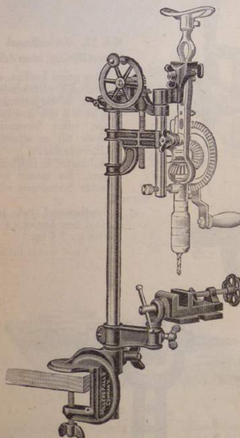
N:o 20. Amerikansk Bröstborrställning, utan bröstbör
