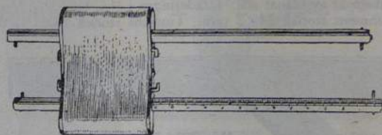
N:o 100. Ritsmått Dubbelt. Extra prima svenskt fabrikat. Genom ett enkelt handgrepp inställas önskade mått snabbt och med undvikande av alla kil- och skruvanordningar. Graderad i mm. och eng. tum. Anslag av lövträ. Beslag och ritsstänger av aluminium. Med ställbara ritspetsar. Graderat upp till 140 mm. Längd 21½ cm.
