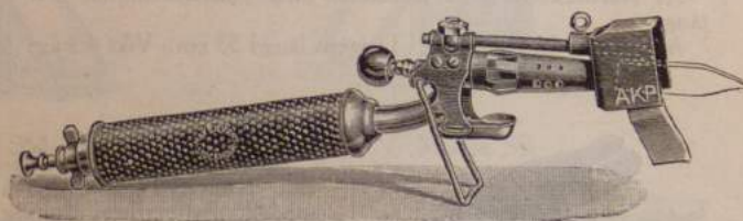
N:o 75. Lödkolv för bensin (gasolja)
