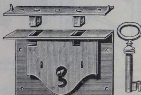
N:o 103. Kistlås med siffernyckel
