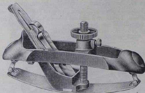
N:o 020. Rundhyvel »Kunz», med dubbelt järn
