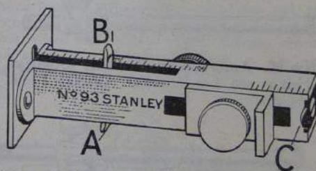
N:o 93. Amerikanskt Ritsmått »Stanley» Helt av stål, fint förnicklat. Graderat i mm. Speciellt avsett för dörr- och fönstergångjärn etc. Längd 9½ cm.
