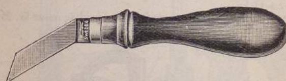
N:o 10. Träsniderikniv, Eskilstuna Extra prima kvalitet (E. A. Berg). Bladets längd 50 mm.
