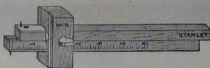
N:o 71. Amerikanskt Ritsmått »Stanley» Dubbelt. Av polerad bok med mässingsbeslag. Graderat i mm. Längd 16½ cm.
