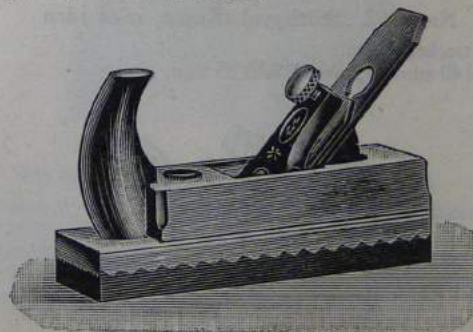
Original »Ulmer» Reform Putshyvel, med dubbelt järn
