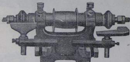
N:o 20. Smärgelslipmaskin
