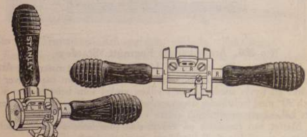
N:o 67. Amerikansk Universal-Spånhyvel »Stanley», med järn
