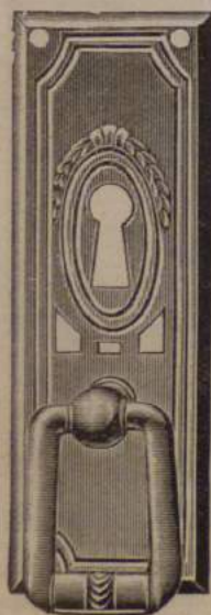
Ringhandtag Av blankpolerad mässing. N:o 469. Utan nyckelhål. Höjd 94 mm. N:o 0469. Med nyckelhål. Höjd 94 mm.
