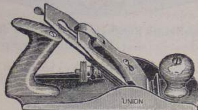
Amerikanska Putshyvlar »Union», med dubbla järn
