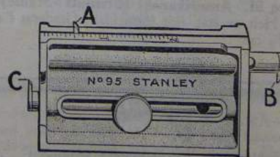
N:o 95. Amerikanskt Ritsmått »Stanley» Av stål, fint förnicklat. Graderat i mm. Speciellt avsett för dörr- och fönstergångjärn etc. Längd 7½ cm.
