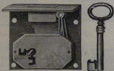
N:o 101. Infällslås med siffernyckel
