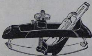
N:o 20. Amerikansk Rundhyvel »Stanley», med dubbelt järn
