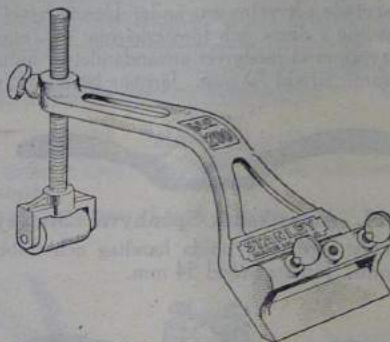
N:o 200. Amerikanskt Slipstöd »Stanley»
