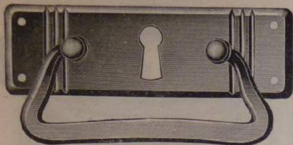
Handtag av blankpolerad mässing N:o 308. Utan nyckelhål. Längd 95 mm. » 0308. Med » » 95 »
